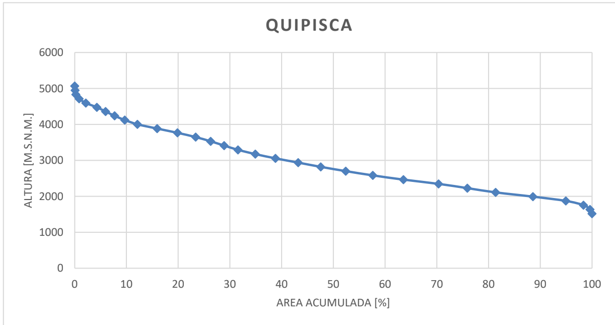
Figura 1 -3 Curva Hipsométrica Quebrada Quipisca.
