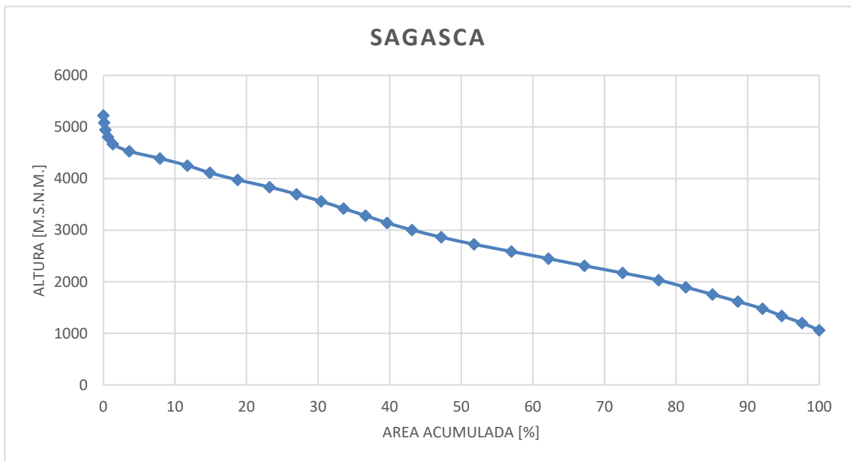
Figura 1 -4 Curva Hipsométrica Quebrada Sagasca.
