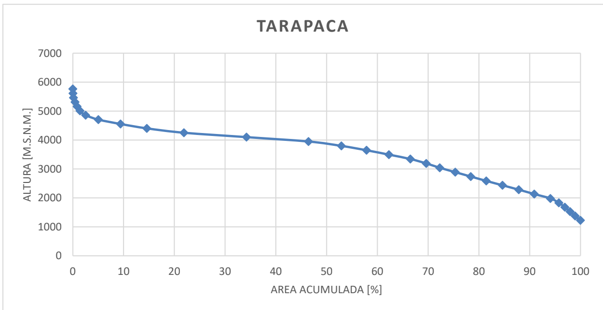
Figura 1 -2 Curva Hipsométrica Quebrada Tarapacá.
