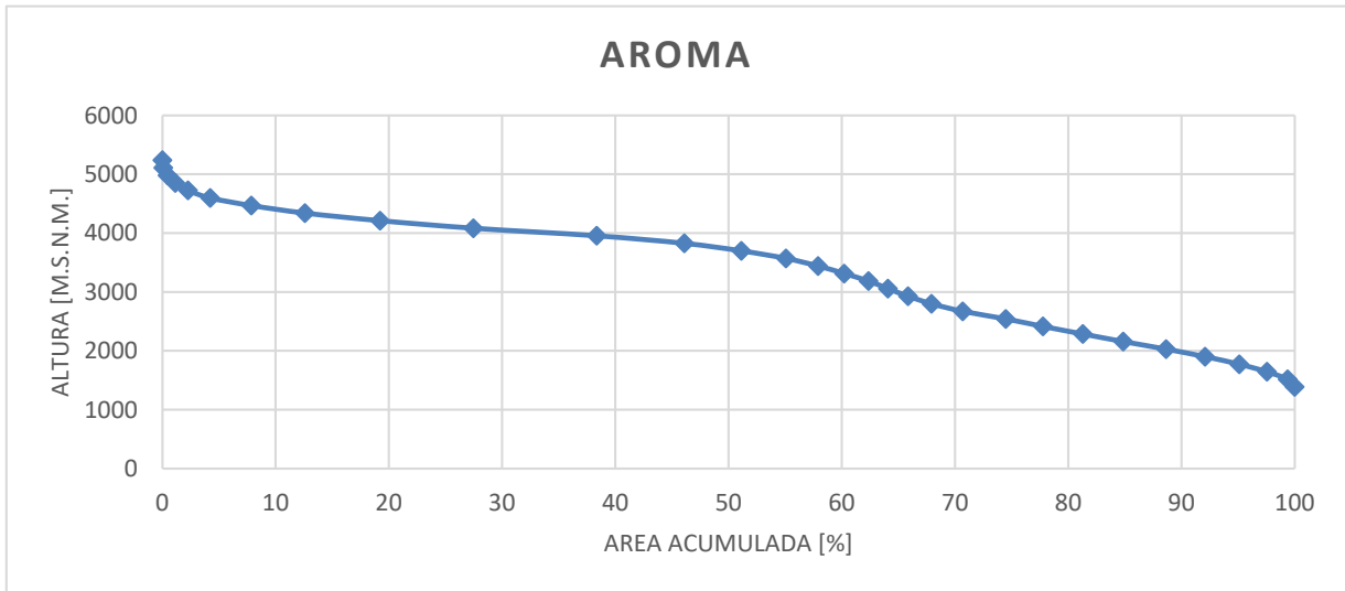
Figura 1 -1 Curva Hipsométrica Quebrada Aroma.
