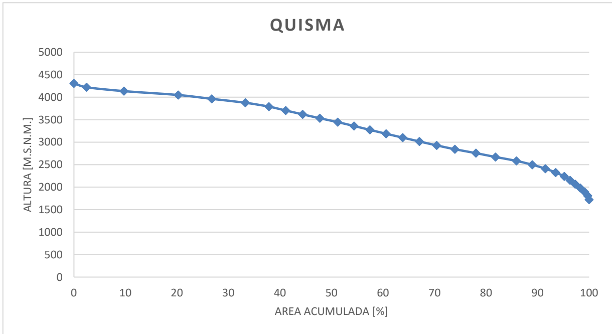
Figura 1 -5 Curva Hipsométrica Quebrada Quisma.
