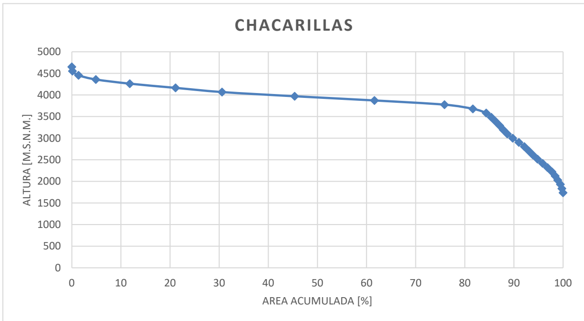
Figura 1 -6 Curva Hipsométrica Quebrada Chacarillas.
